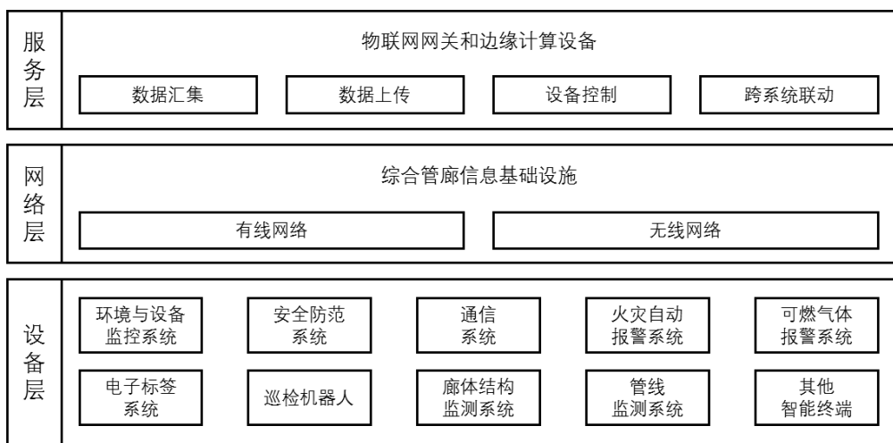
图 A-2 综合管廊物联网总体架构图
